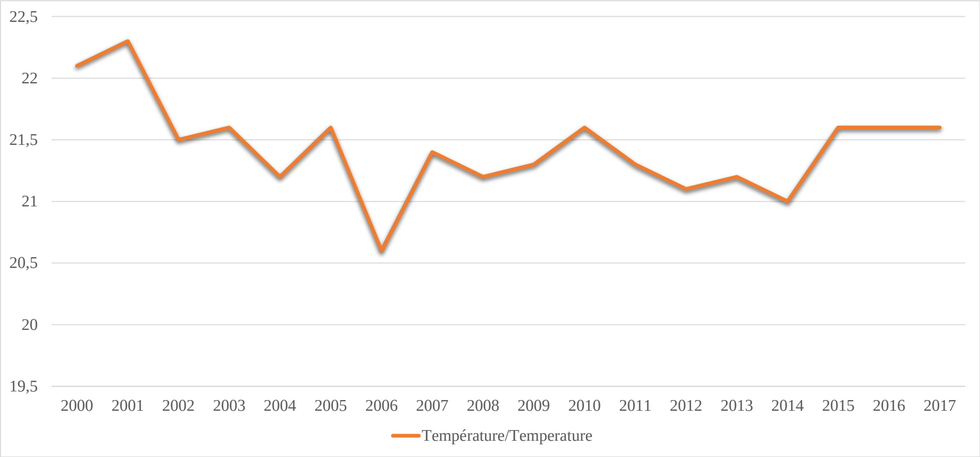
Variation des moyennes annuelles des températures de Ngaoundéré entre 2000 et 2017/ Variation of annual average temperatures of Ngaoundéré between 2000 and 2017
